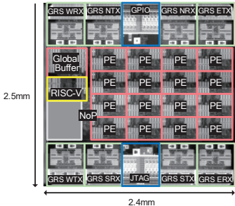
Fig. 5: Die micrograph.
