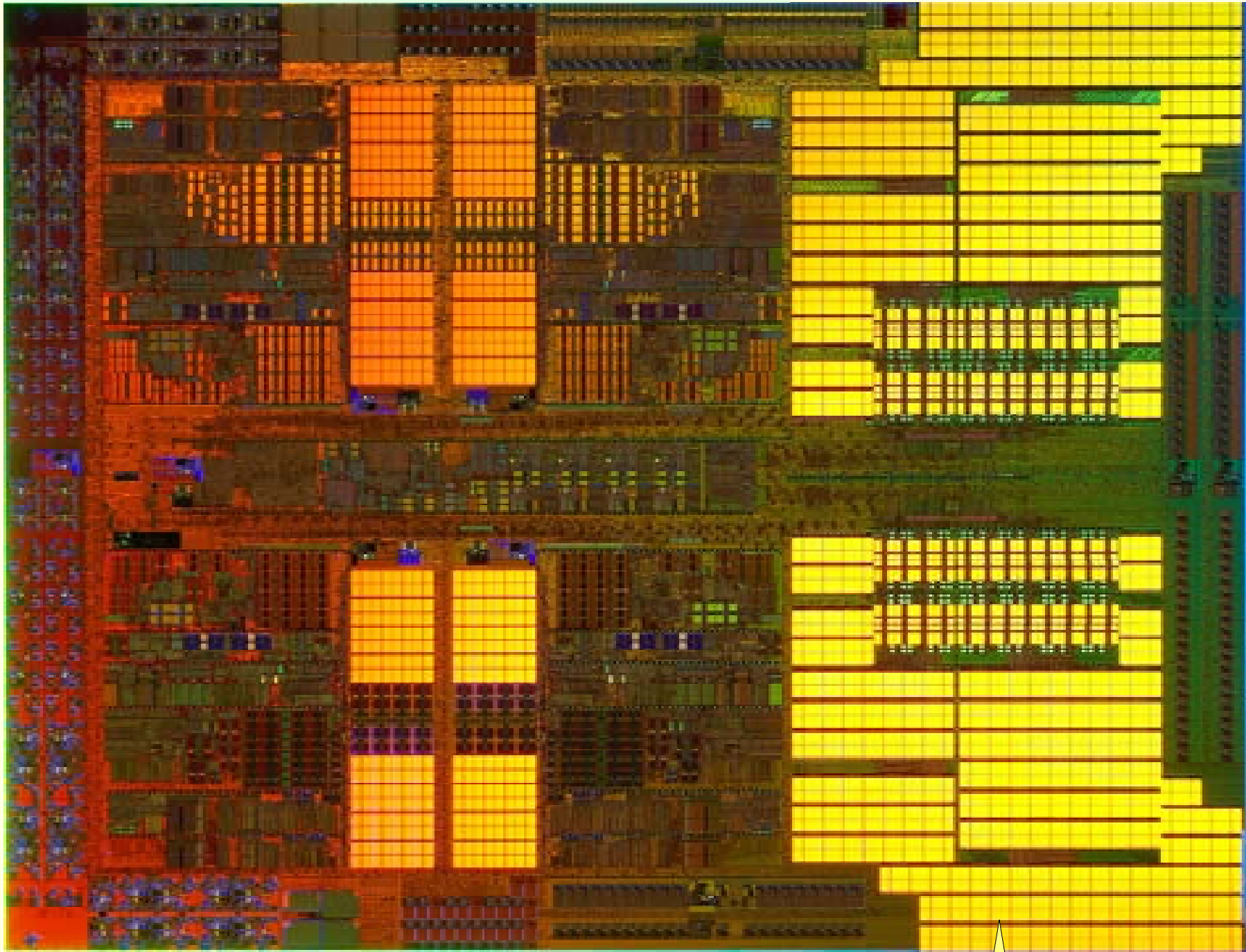
4 Core(0.5MB L2) + 6MB L3
