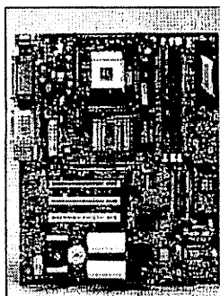
AOpenのAX4B-533 Tube。上部3分の2を見れば普通のATXマザーだが、下部がちょっと異様な光景 デジタルとアナログの融合を成功させたことを示す「Tube Sound TECHNOLOGY」のエンブレム
