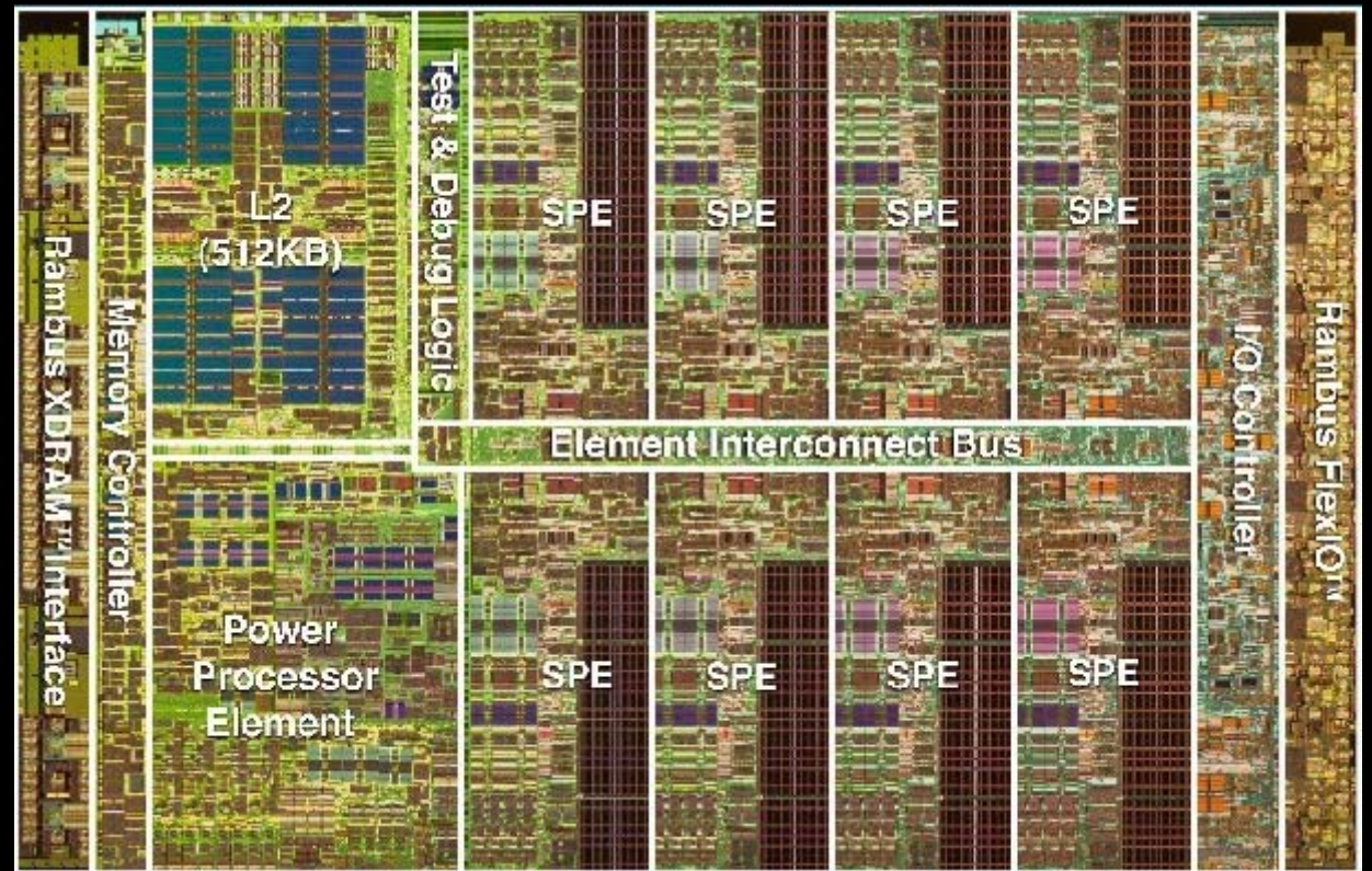
90nm Cell B.E.
