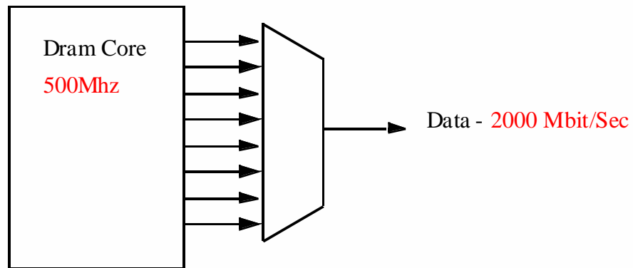
GDDR4 Prefetch 8
