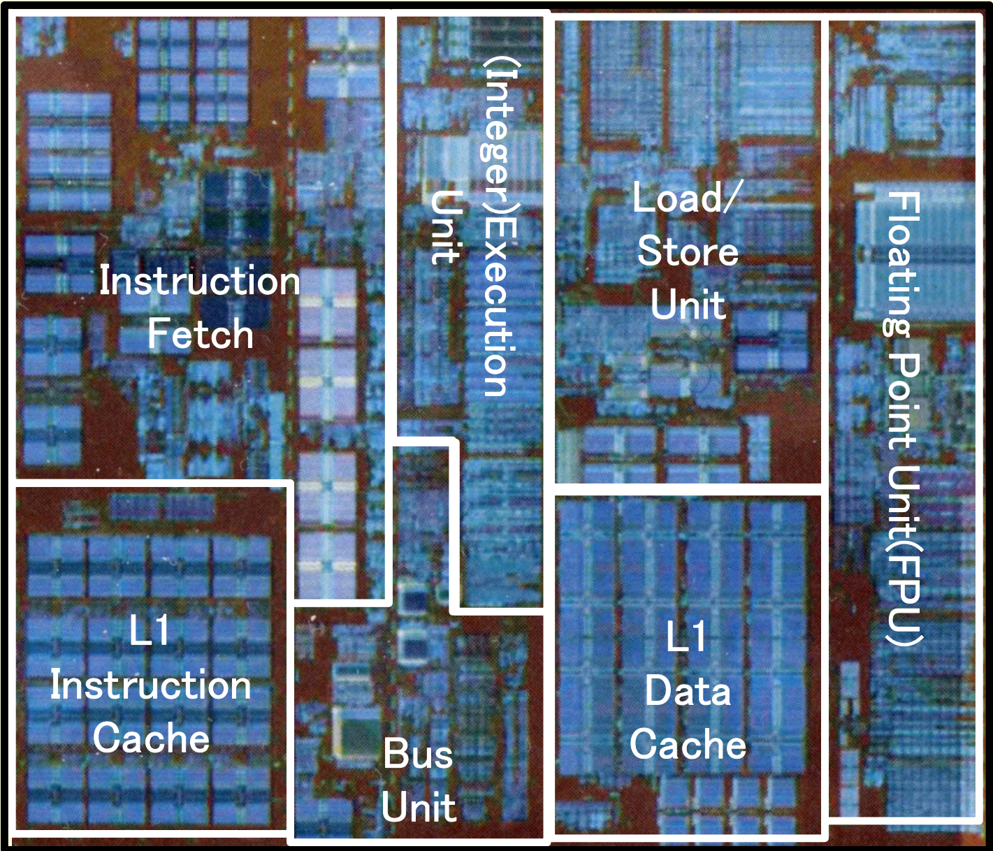
Rev. G? K8 CPU core (AMD Briefing April '06)
