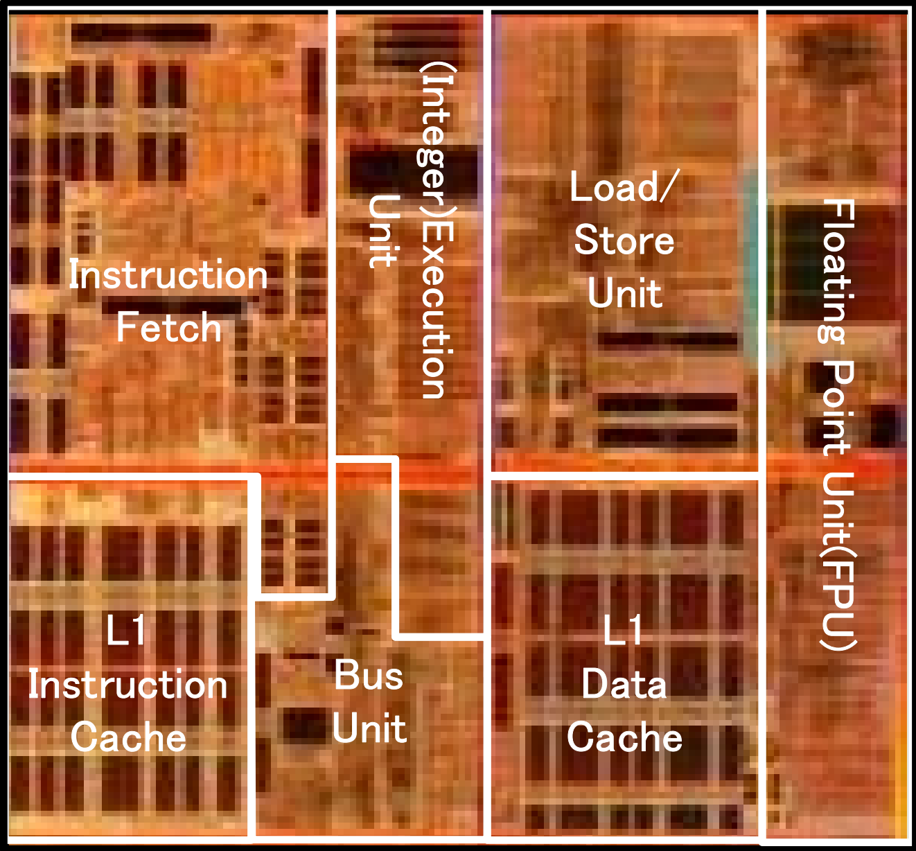
Rev. F K8 CPU core (ISSCC 06)
