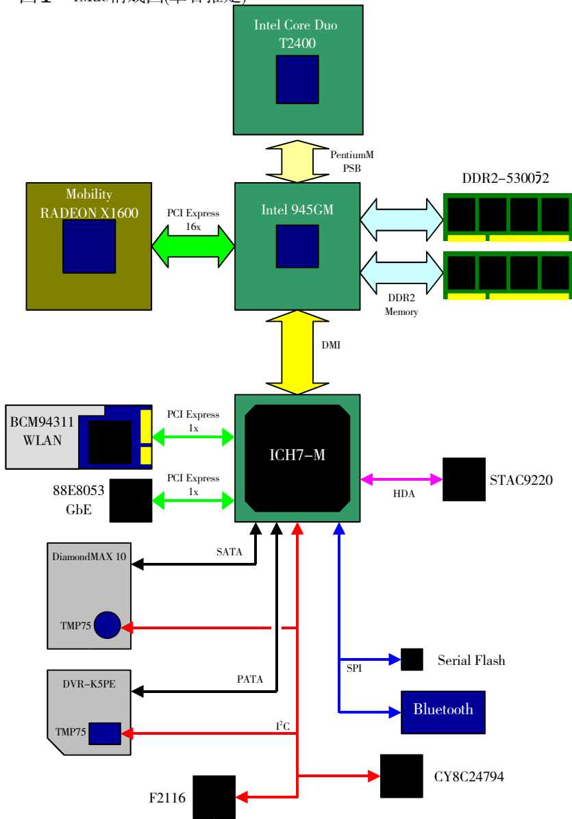
图1：iMac構成図(筆者推定)
